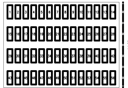
PREDISPOSIZIONE FOSSE CAMPO N. 15 SCALA 1:100
